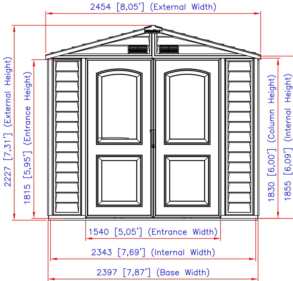
Elevation
